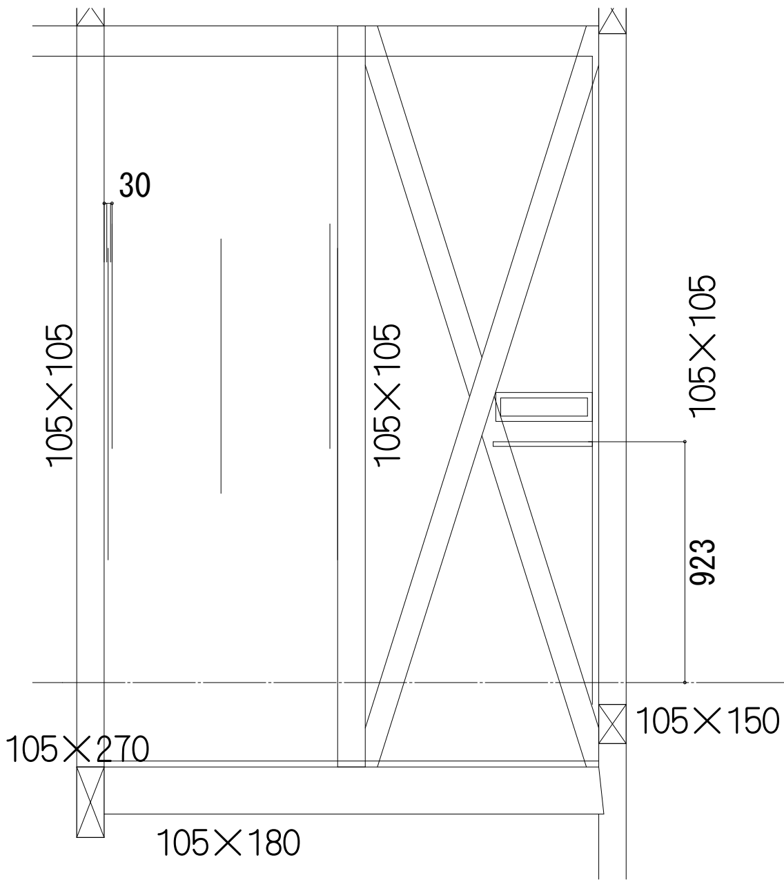
35面 軸組図 S:1/20
