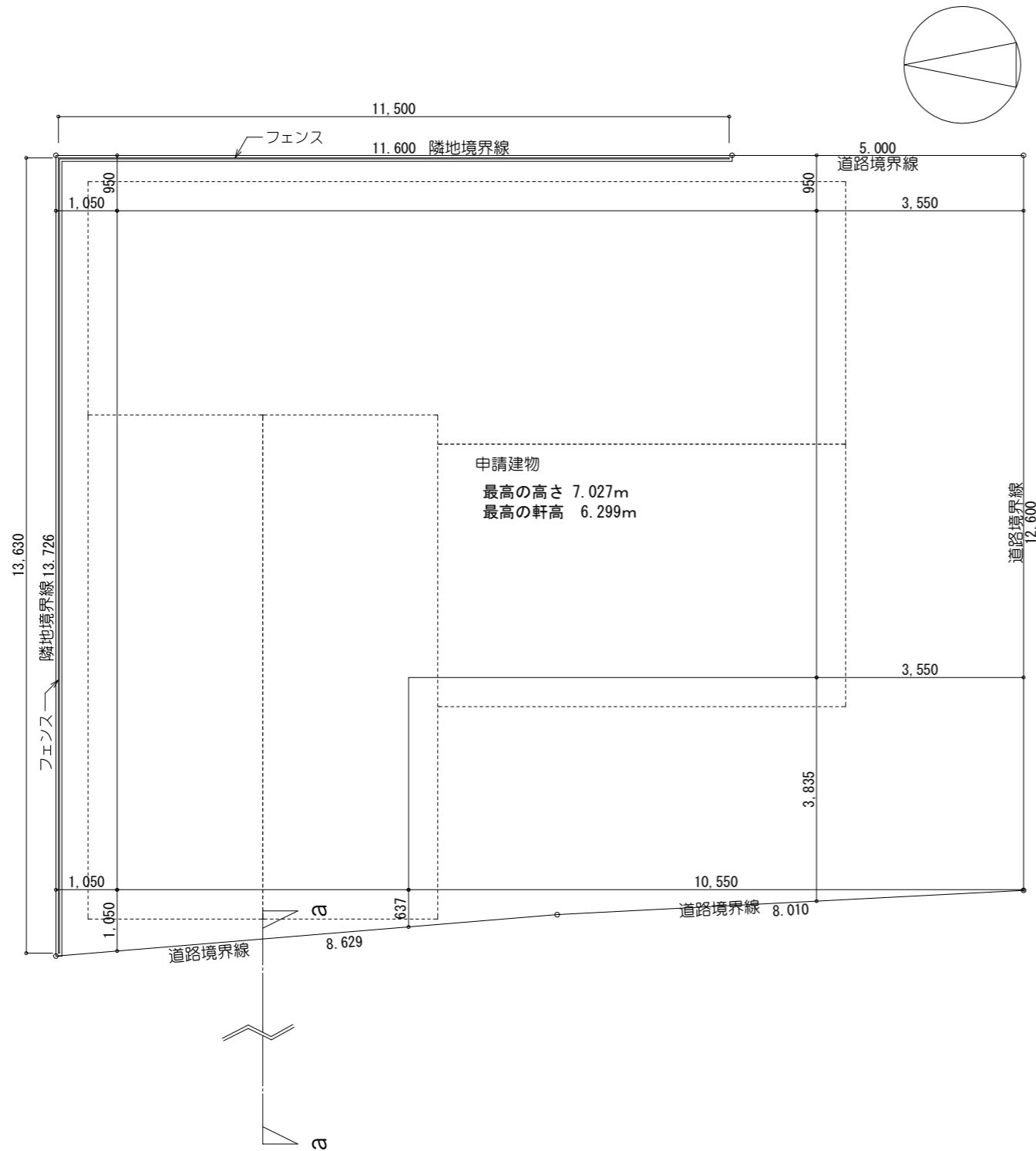
配置図 S:1/100
