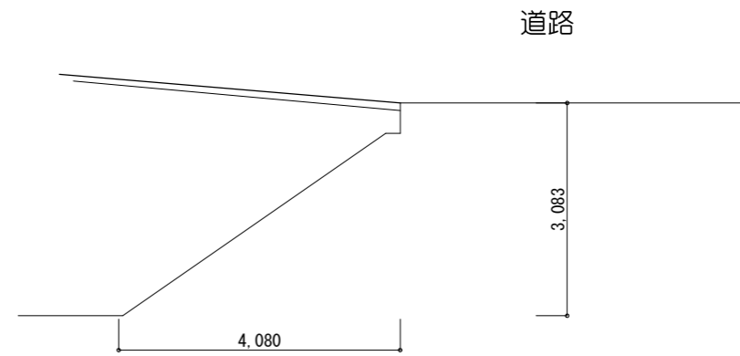
a-a断面図 1/100
