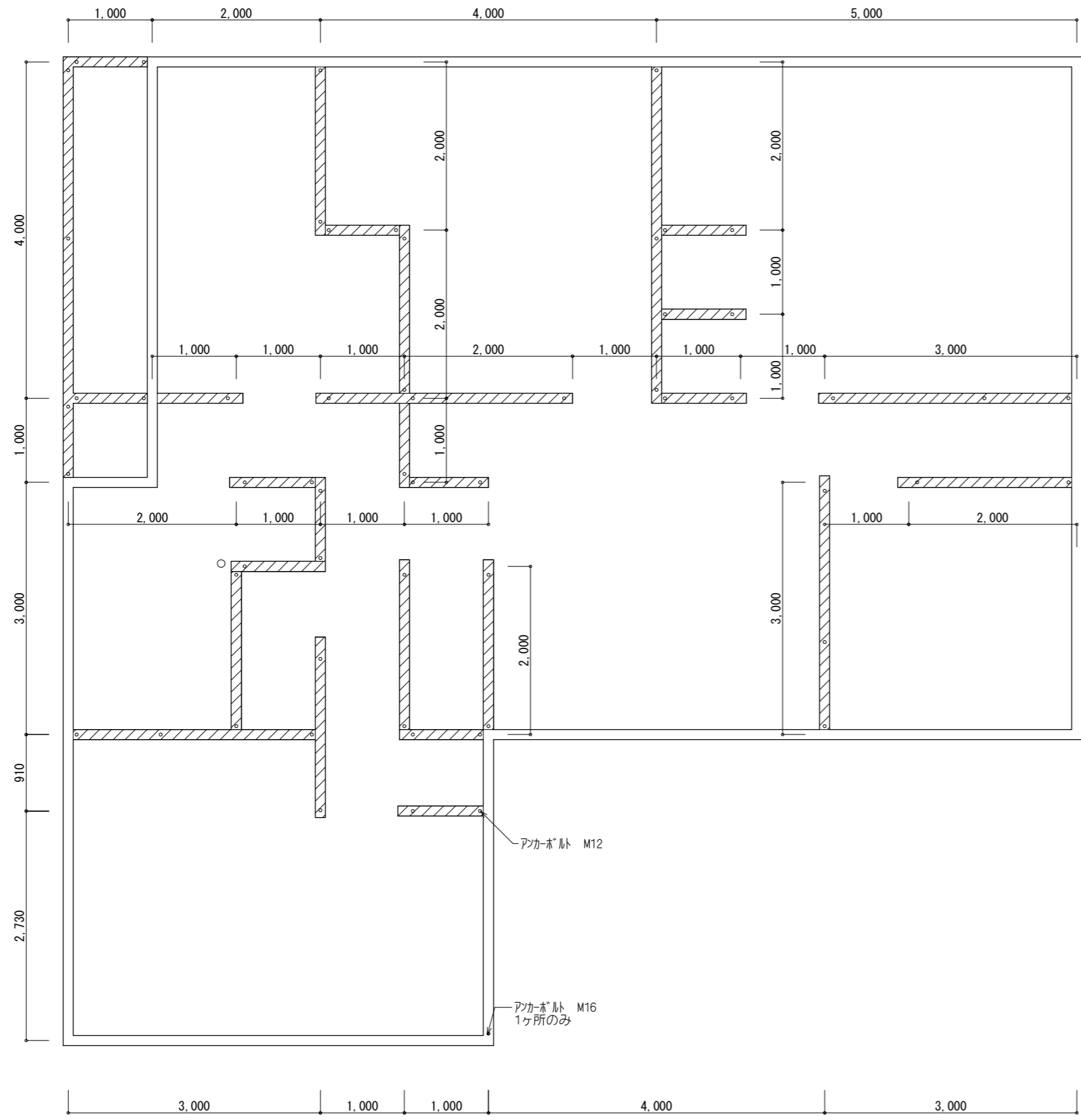
基礎伏図 S:1/60
