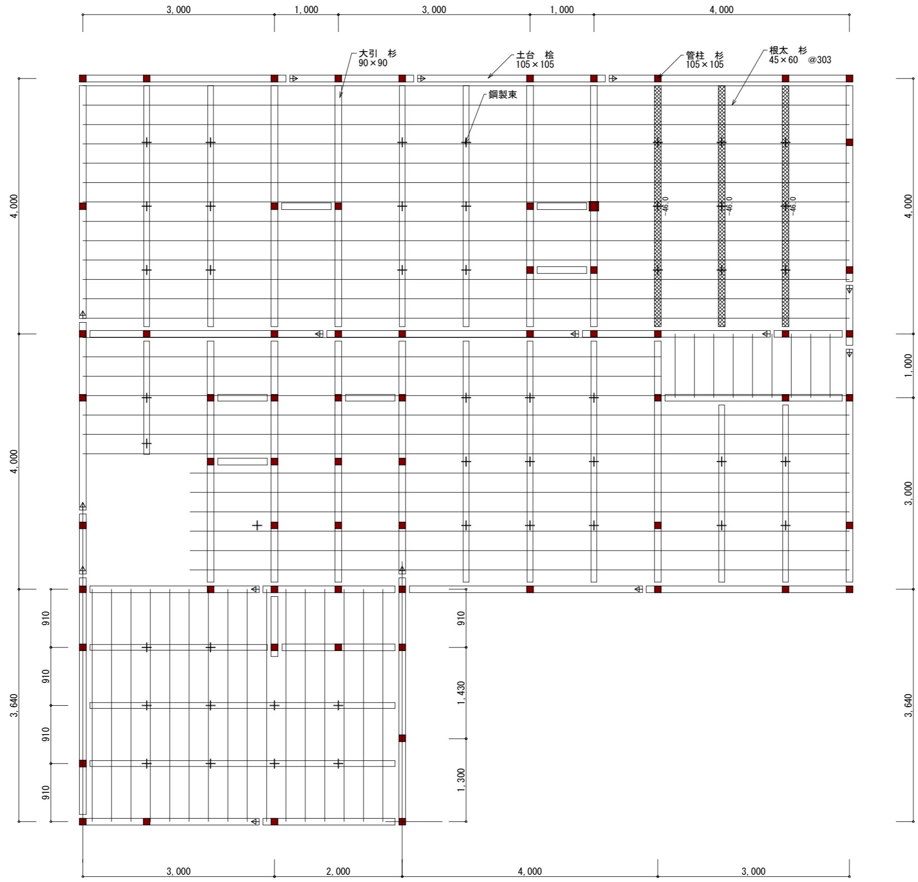
1階 床伏図 S:1/60
