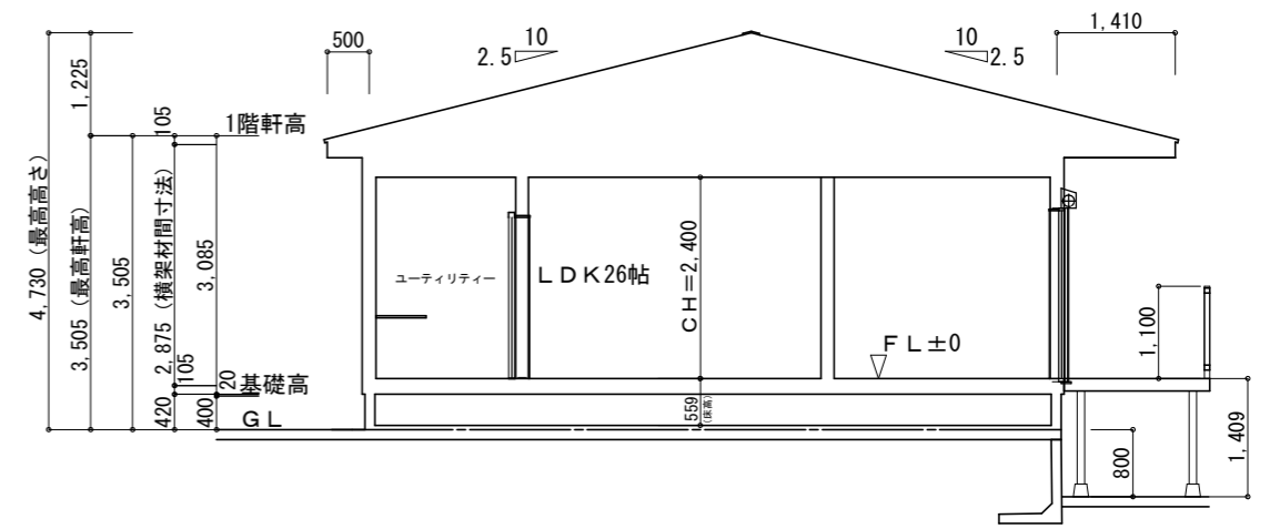
断面図 1/100
