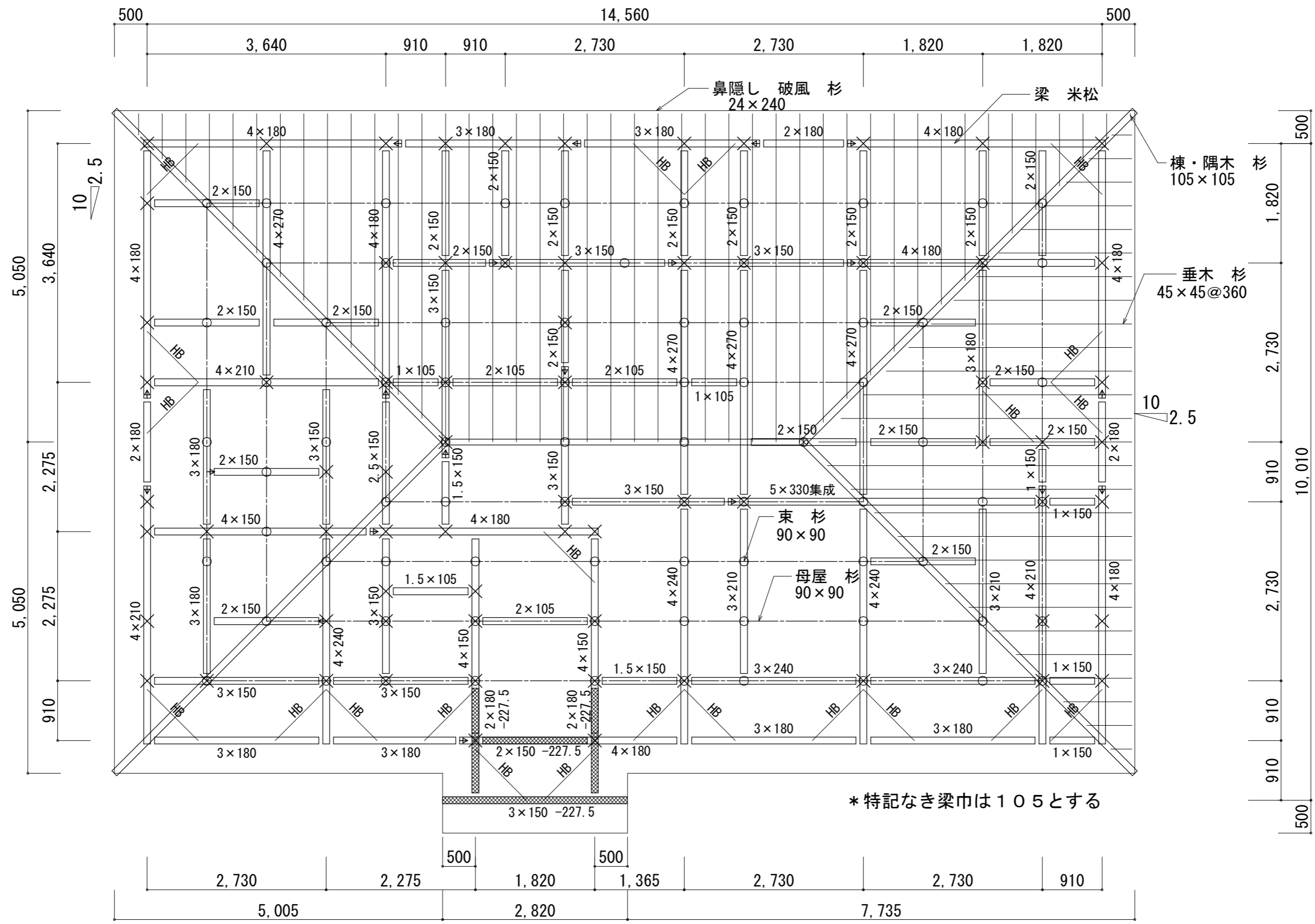
小屋伏図 S:1/60
