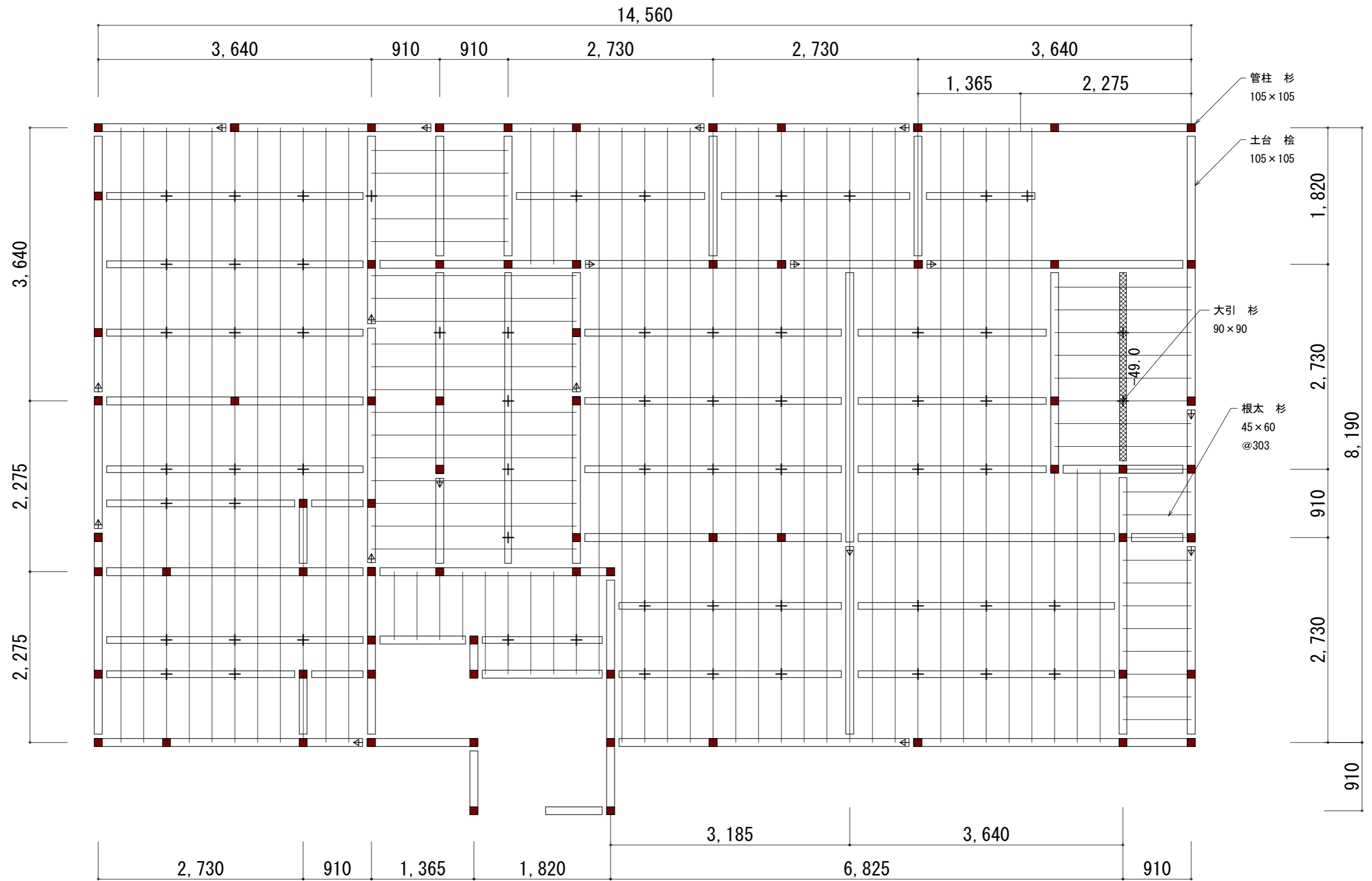
1階 床伏図 S:1/50
