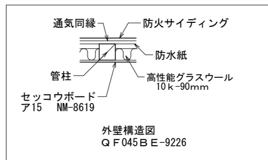
断面図 1/100
