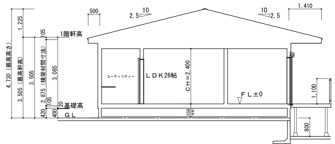
断面図 1/100
