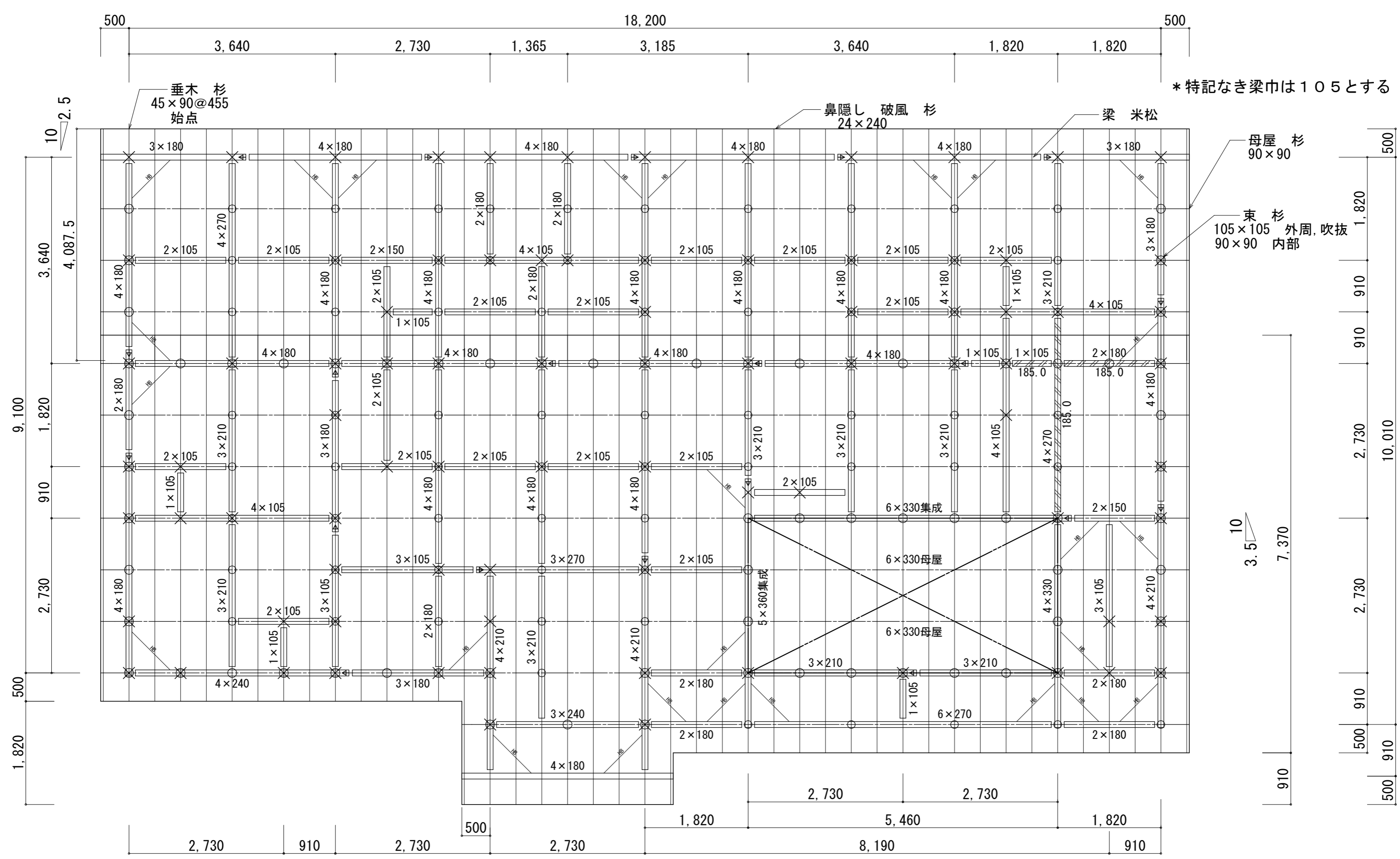
小屋伏図 S:1/60
