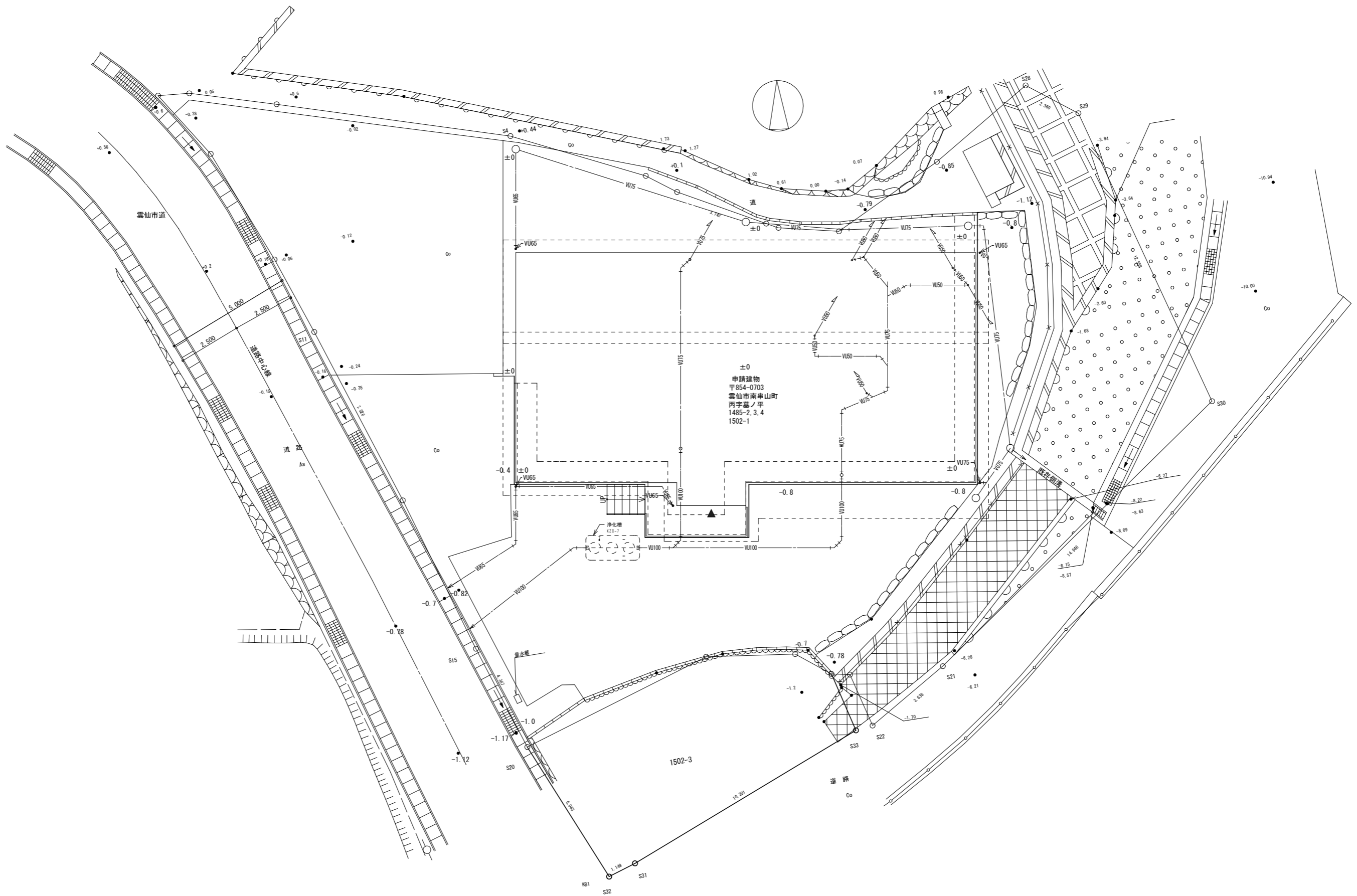
配置図 S:1/150
