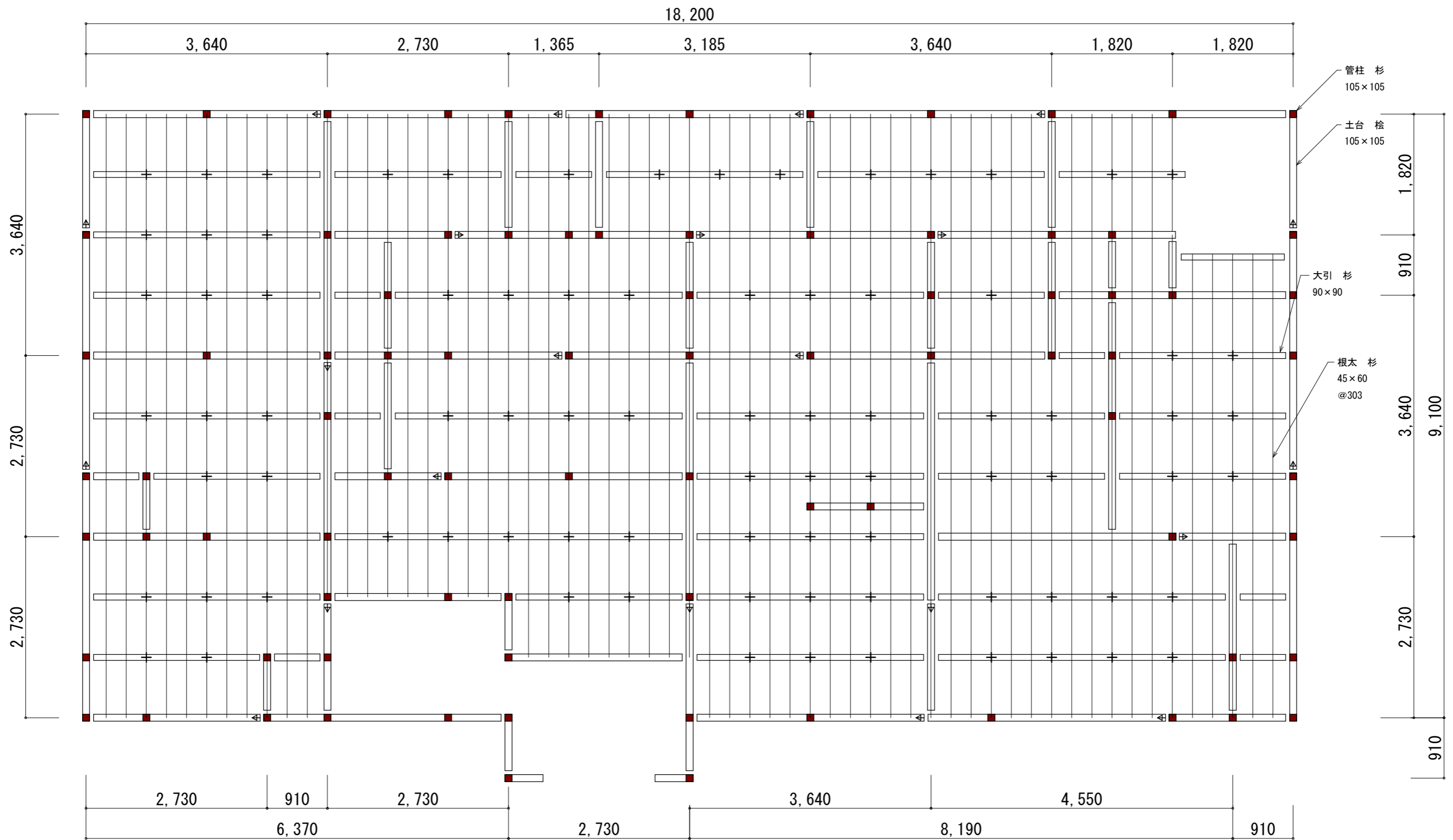
1階 床伏図 S:1/60
