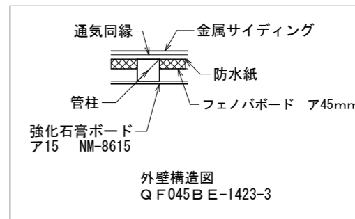
断面図 1/100
