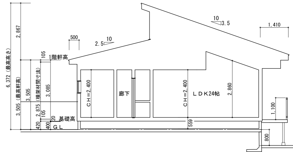
断面図 1/100
