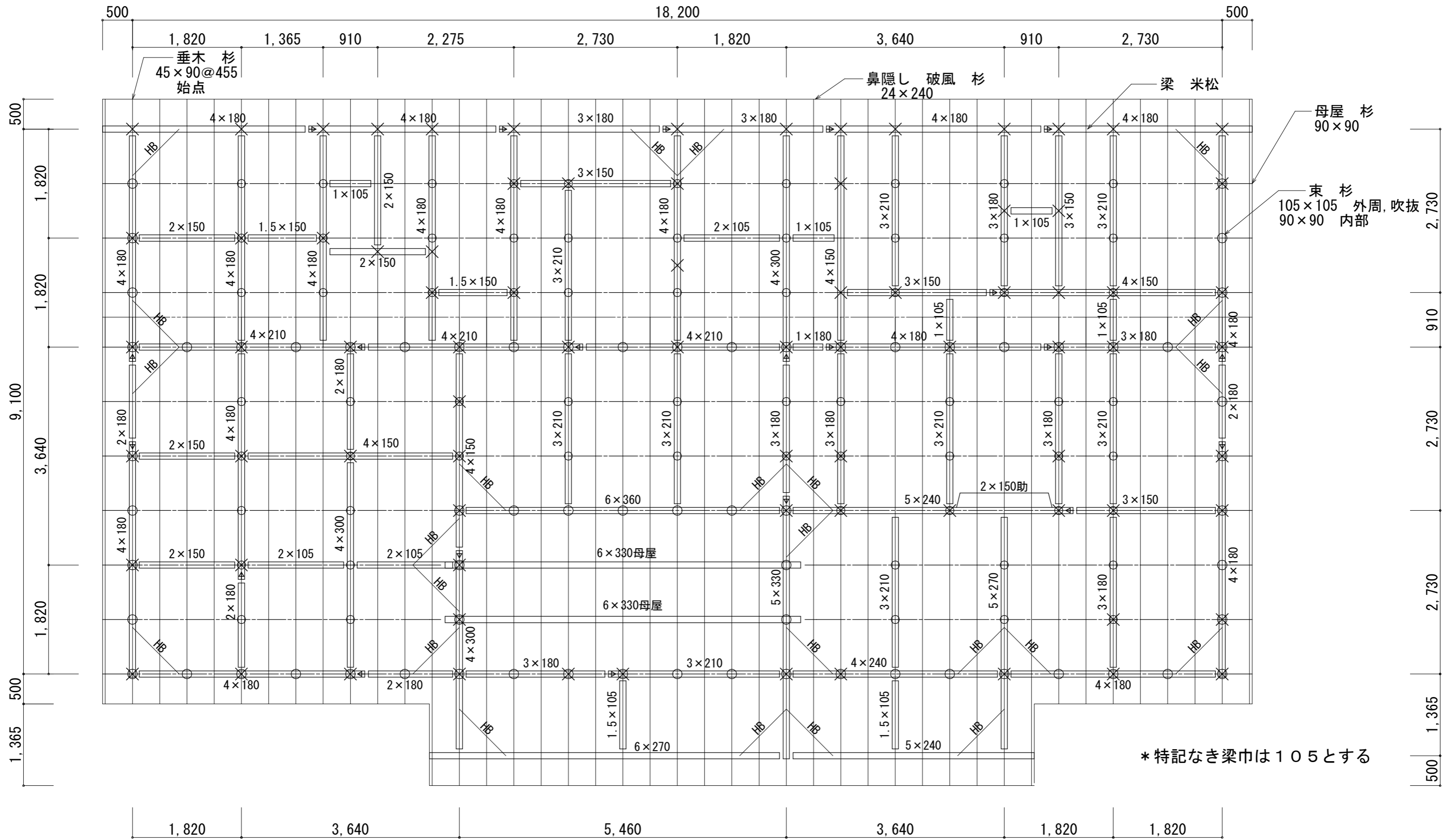
小屋伏図 S:1/60
