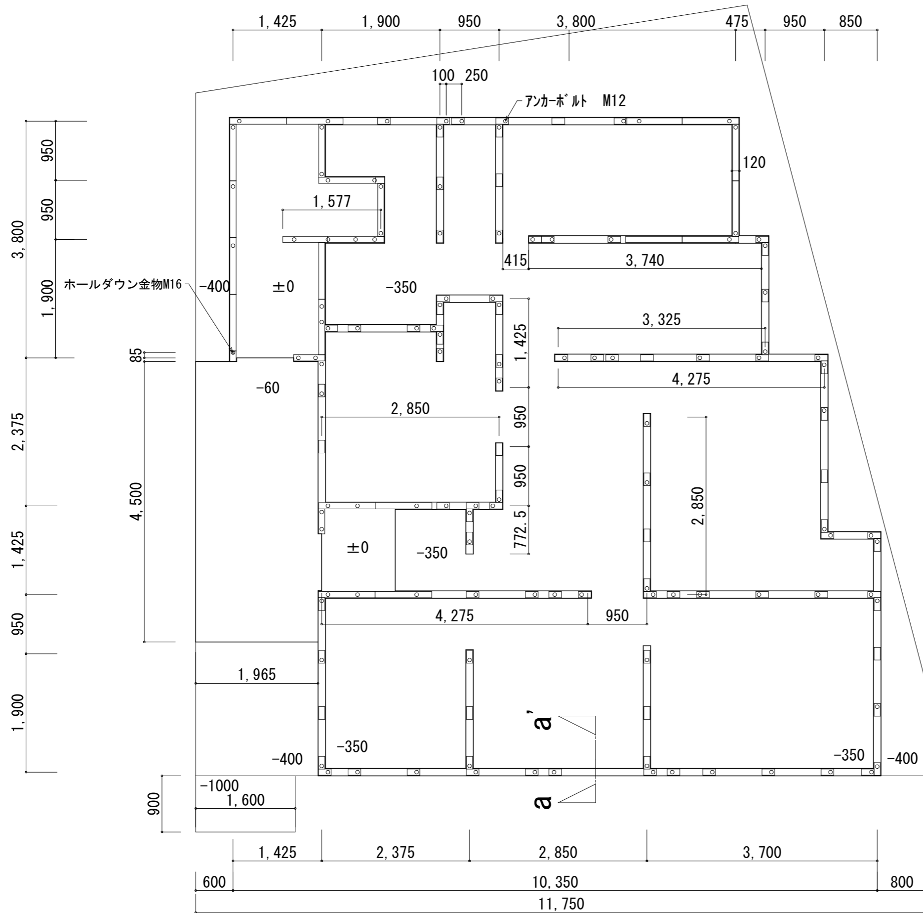
基礎伏図 S:1/60
