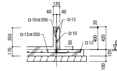
べた基礎断面
