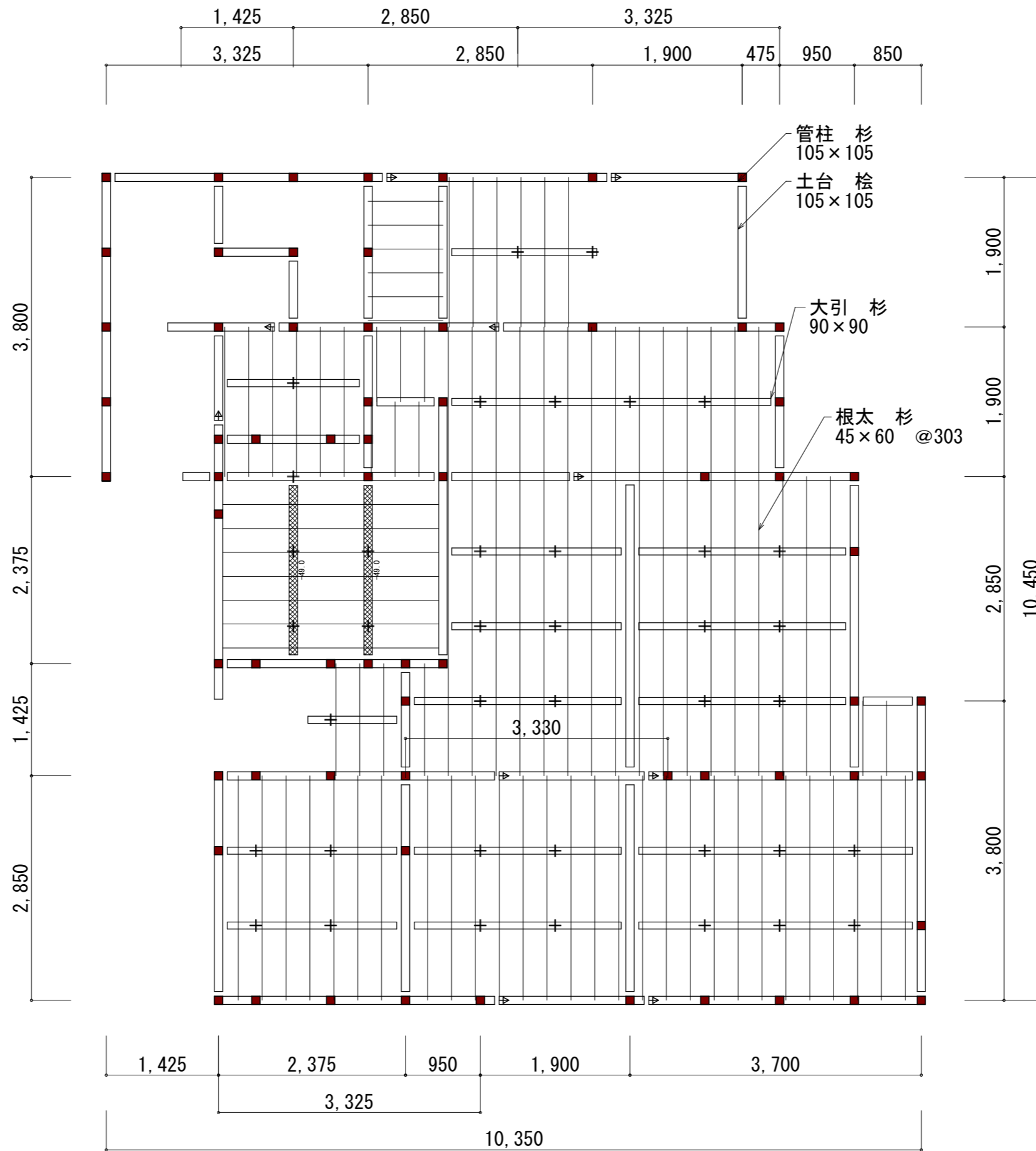
1階 床伏図 S:1/60
