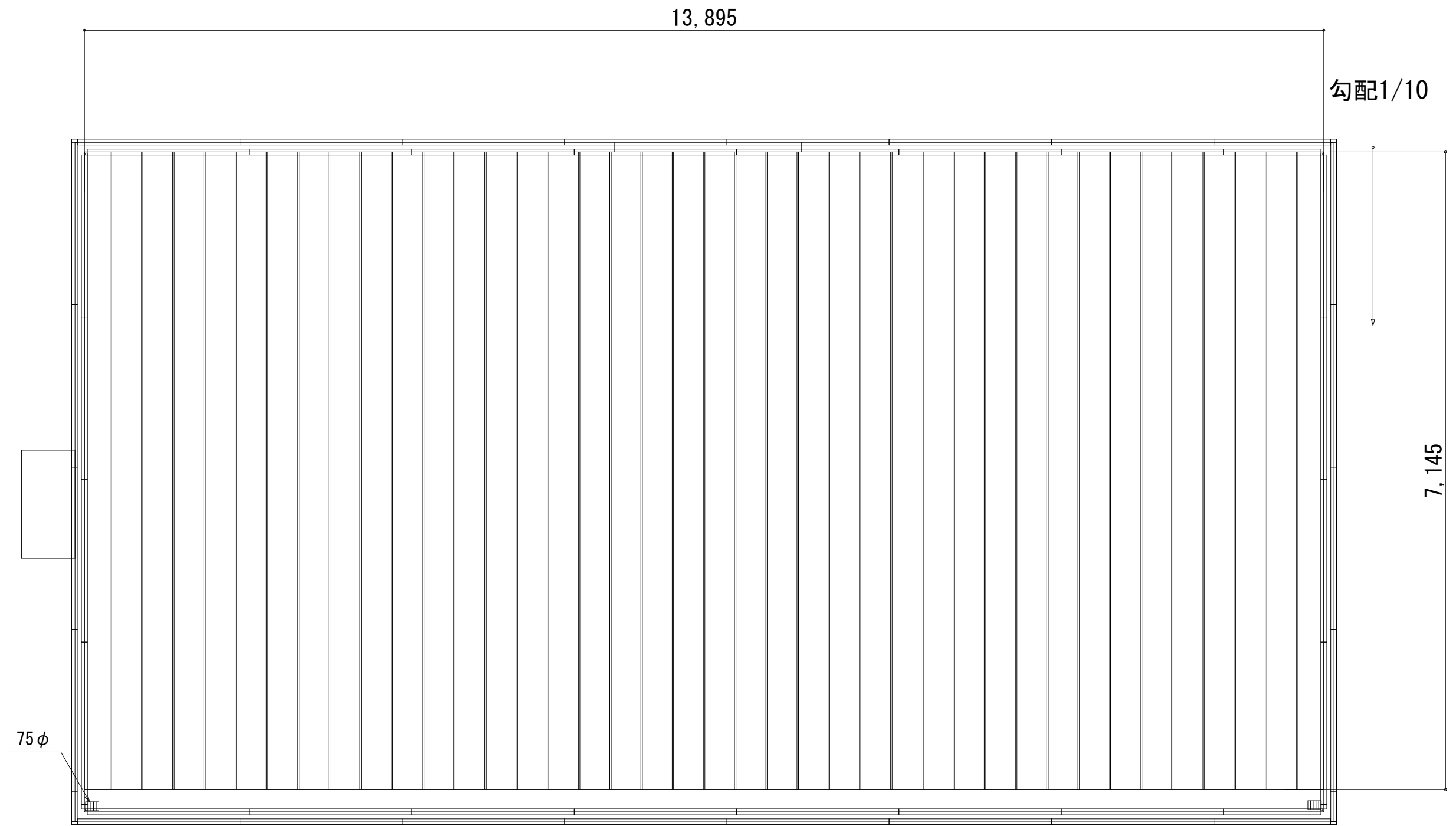
2階 屋根伏図 S:1/50
