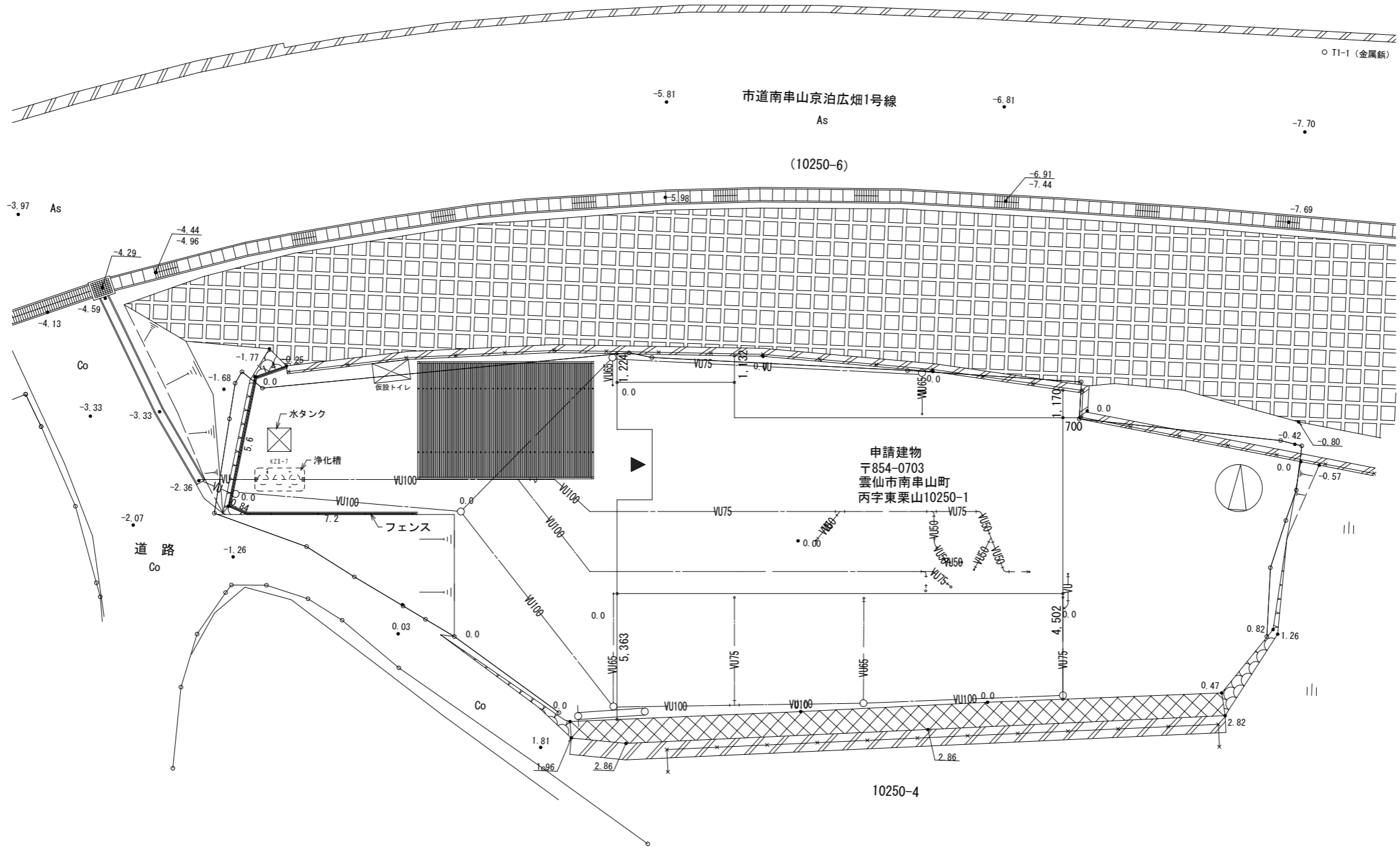
配置図 S:1/200
