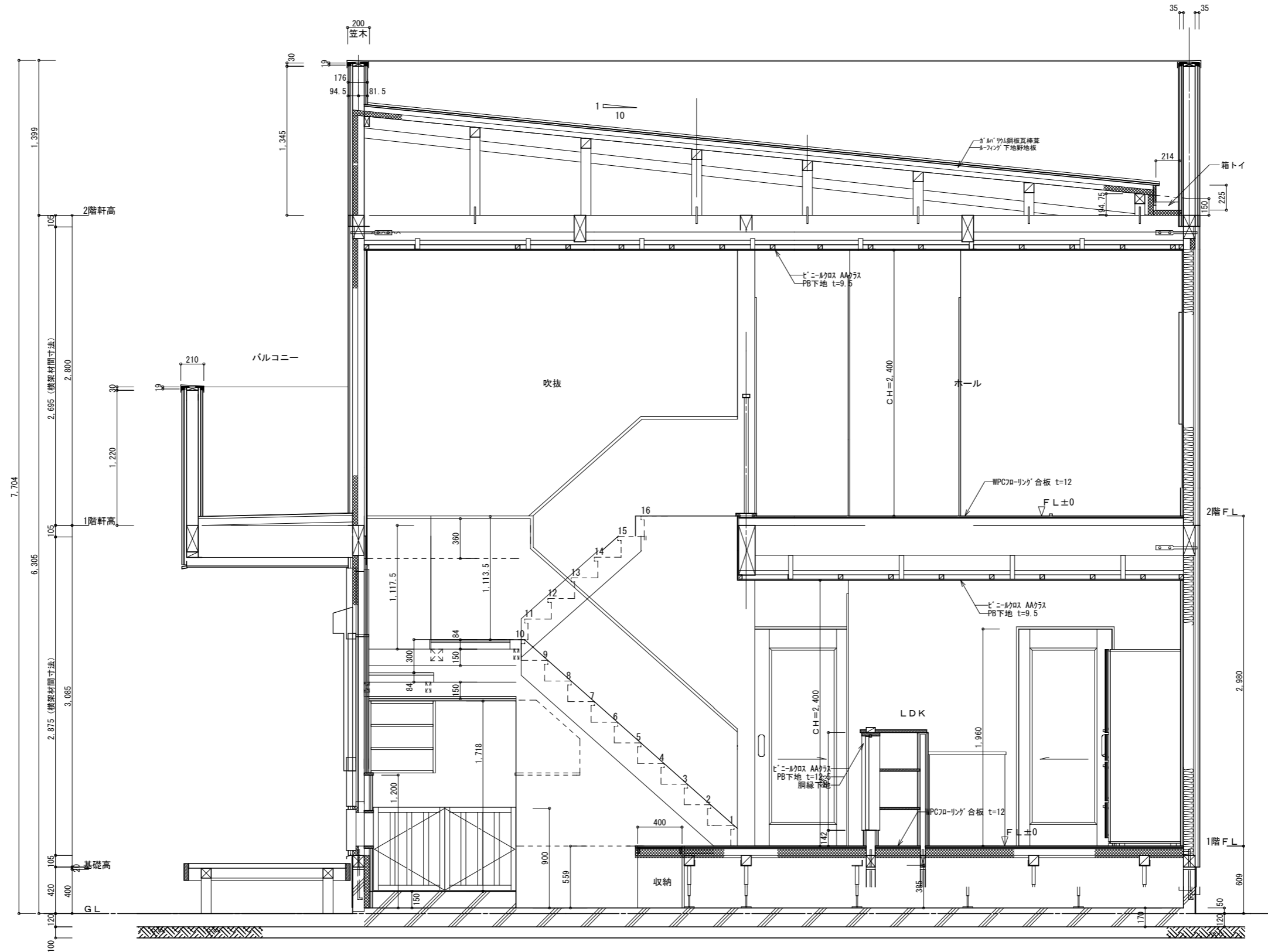
3面 矩計図 S:1/40
